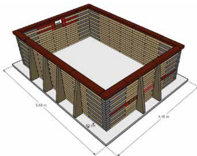
POSE HORS-SOL/SEMI-ENTERRÉE (1/3 ENTERRÉE) 12X RENFORTS OBLIGATOIRES
