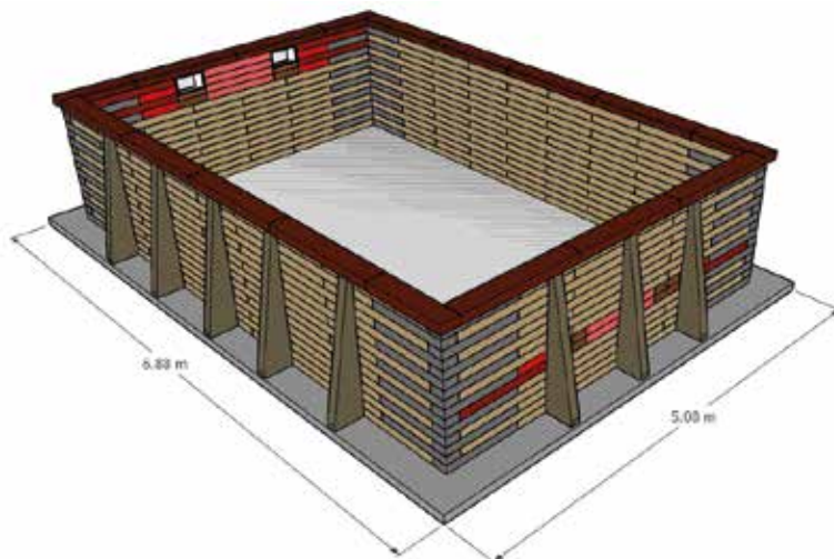
POSE HORS-SOL/SEMI-ENTERRÉE (1/3 ENTERRÉE) 16 X RENFORTS OBLIGATOIRES
