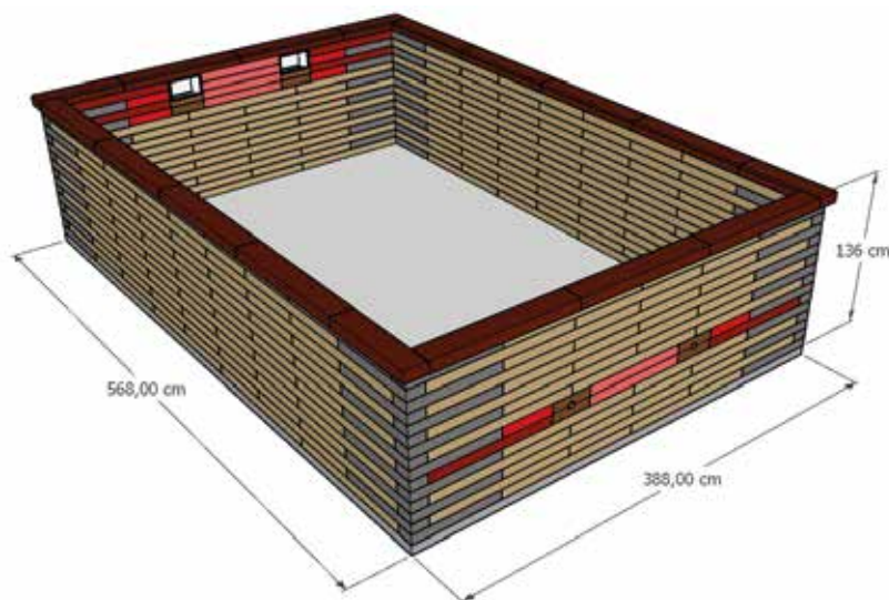
POSE ENTERRÉE/SEMI-ENTERRÉE (2/3 ENTERRÉE)
