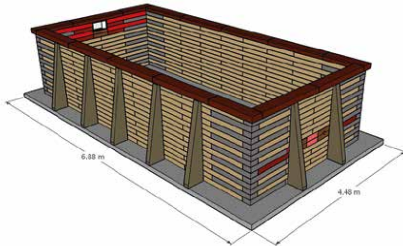
POSE HORS-SOL/SEMI-ENTERRÉE (1/3 ENTERRÉE) 14X RENFORTS OBLIGATOIRES
