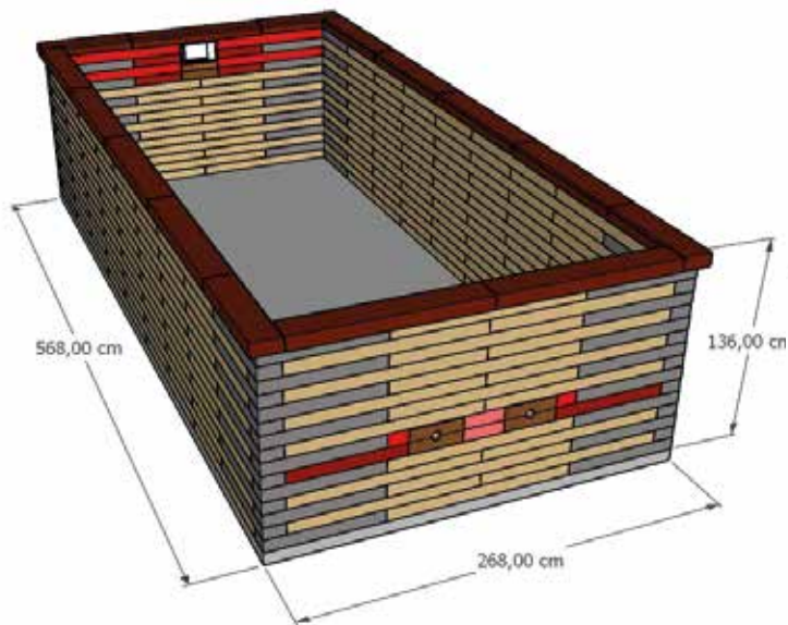
POSE ENTERRÉE/SEMI-ENTERRÉE (2/3 ENTERRÉE)
